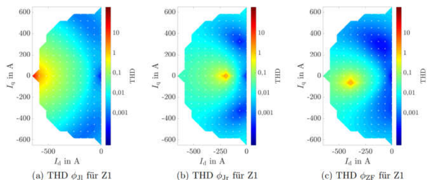
Abb.1. Harmonische Anteile des magnetischen Flusses im Einzelzahn einer permanentmagneterregten Synchronmaschine über den Betriebsbereich
